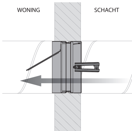
1. Installatierichting voor toevoer.
