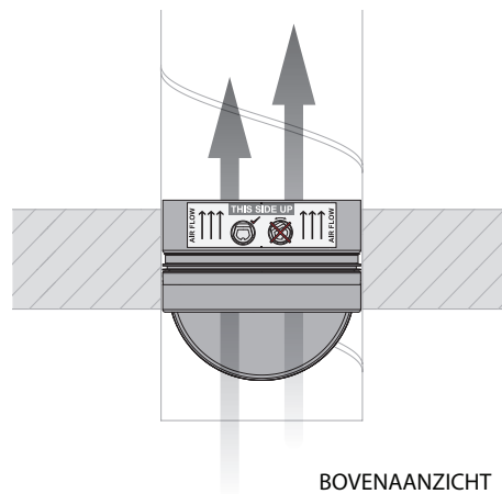
4. Bovenaanzicht.
