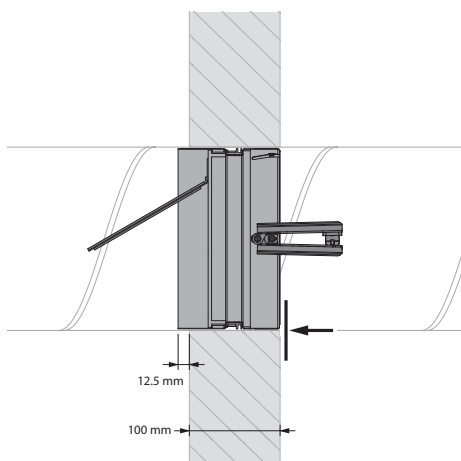
5. Plaatsing t.o.v. compartimentswand.
