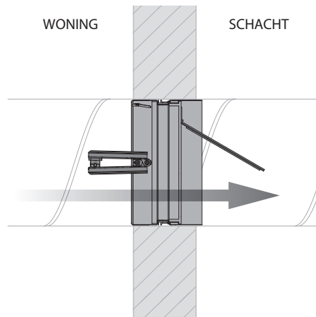
2. Installatierichting voor afvoer.
