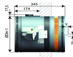
Uitsteken klepblad: 20 mm bij Ø300- 315
