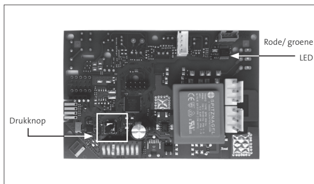
Fig. 1 - Ontvanger printplaat in het toestel
